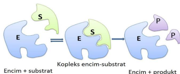
Slika 1: Pri encimsko katalizirani reakciji se molekula substrata pretvori v molekulo produkta. Substrat (S) se mora najprej vezati na encim (E) in tako nastane kompleks encim-substrat (ES), nato poteče reakcija in substrat se pretvori v produkt (P). Kompleks encim-produkt razpade na nespremenjeno molekulo encima in molekulo produkta (Urzi, 2015)
